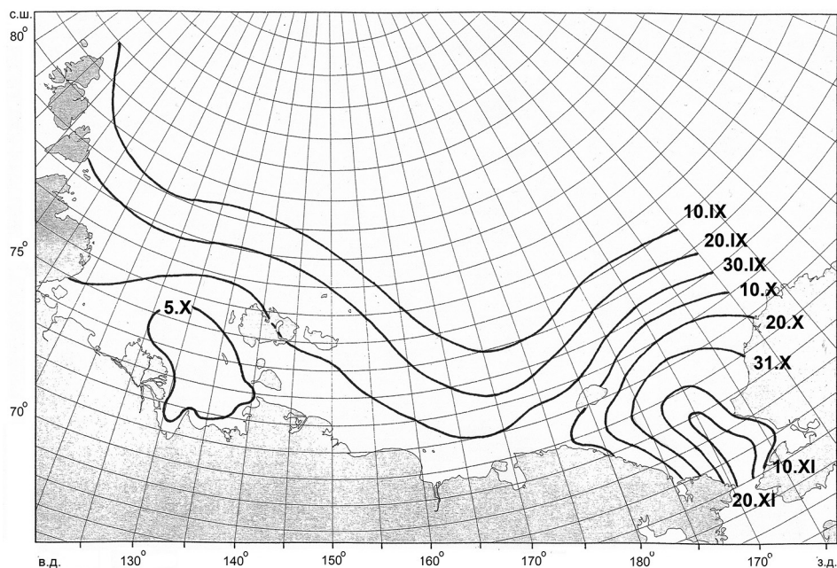
Рис. 1. Карта среднеголетнего распределения изохрон устойчивого ледообразования в восточных арктических морях России в течение 1942–2018 гг.
