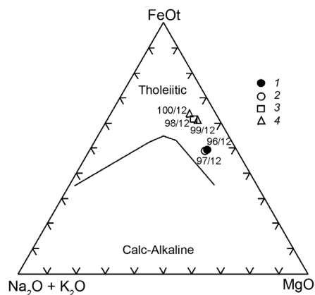
Рис. 5. Диаграмма AFM для габброидов о. Питерман: 1 — габбро темной полосы тонкопослойчатых габбро; 2 — вмещающие габбро; 3 — жильные тела габбронорита амфиболитизированного с порфирированной структурой; 4 — габброиды других участков о. Питерман
