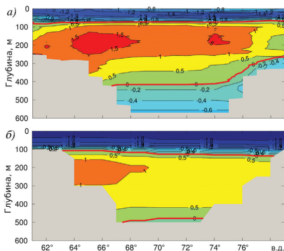
Рис. 8. Распределения температуры на разрезе по 81,5^{\circ} с.ш. в желобе Св. Анны: а — 2000-е гг. по данным наблюдений, б — 1970-е гг. по данным Атласа EWG [33]
